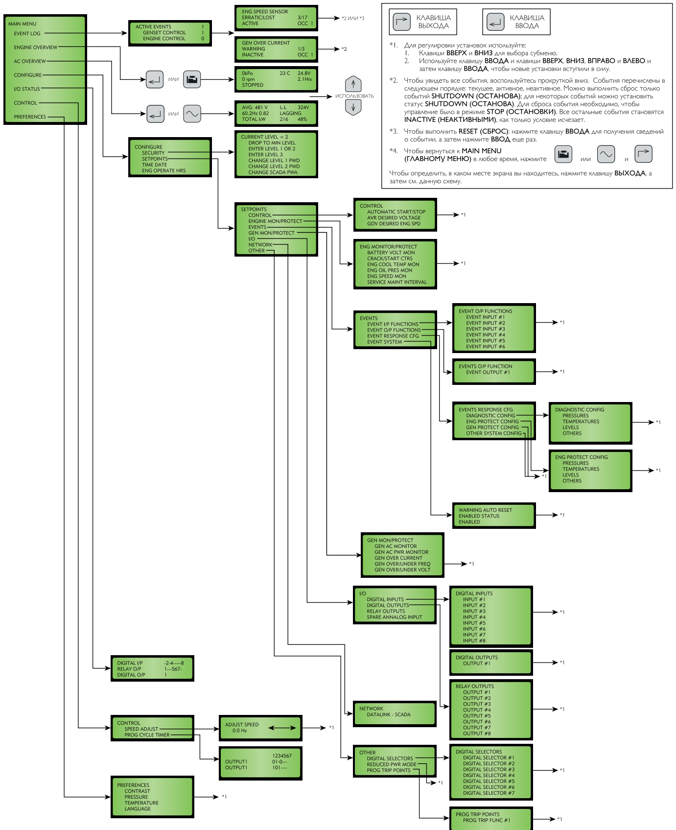
Структура меню управления генераторной установкой PowerWizard 2.0
